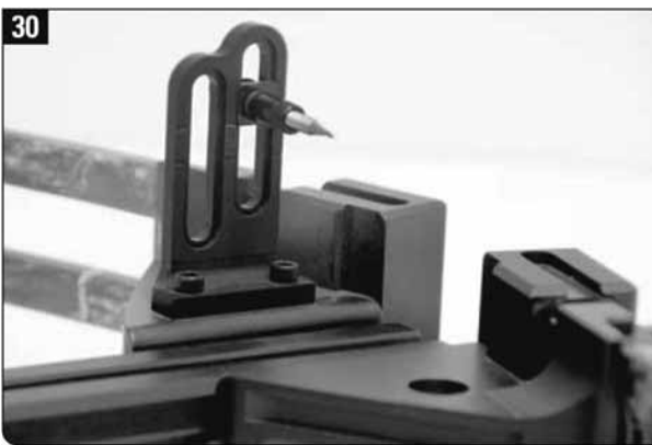
30. Установите намушник с мушкой на левой стороне колодки (для моделей «Titan TL-7» и «Slider»)
