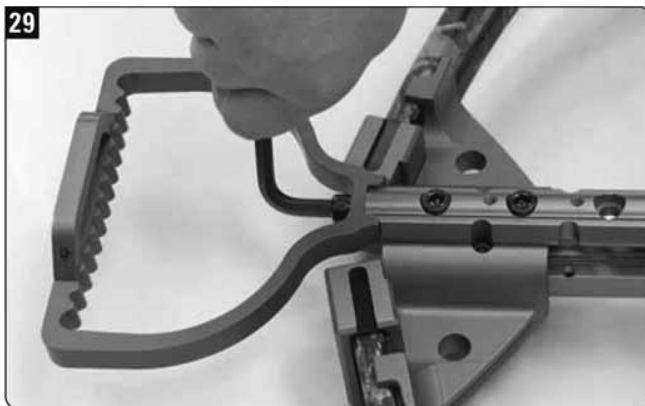
29. Присоедините стремя прямо к нижней части ствола «UL TriLoc»
