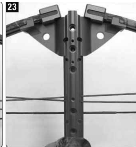
23. Фронтальная часть в «длинной» позиции
