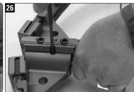
26. Продолжайте прижимать обе части ствола друг к другу, затягивая два более мелких крепежных винта
