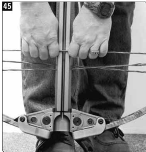
45. Если вы не будете в точности исполнять указания данного руководства во время взведения арбалета и закладки стрелы, вам не удастся добиться высокой кучности при стрельбе
