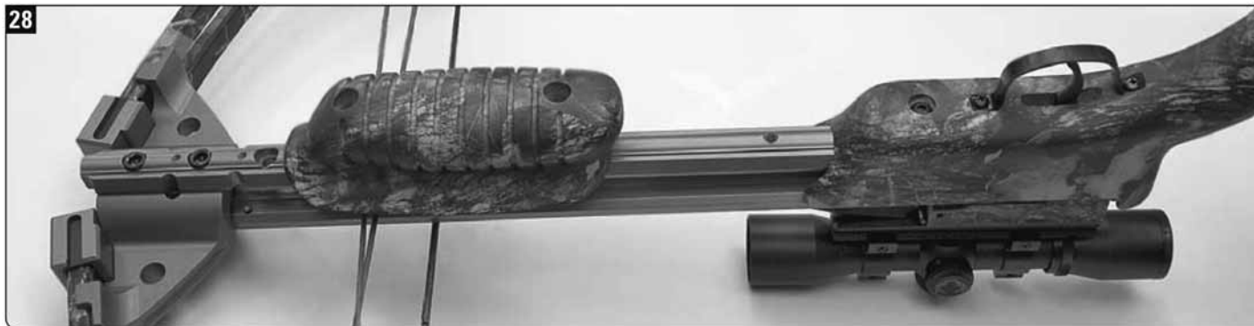
28. Цевье в «длинной» позиции
