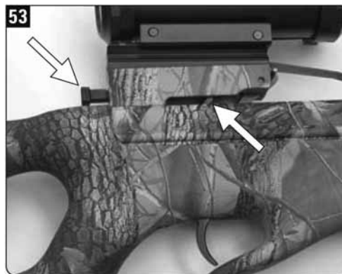
53. Спусковой механизм «RollerTouch» оснащен плунжером и «опускающейся» (или «падающей») защелкой для тетивы
