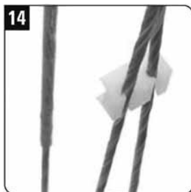
14. Убедитесь, что кабели вошли в соответствующие прорези бегунка
