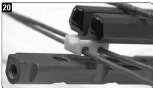
20. Форма желоба на одной из сторон бегунка должна соответствовать профилю нижней части направляющей
